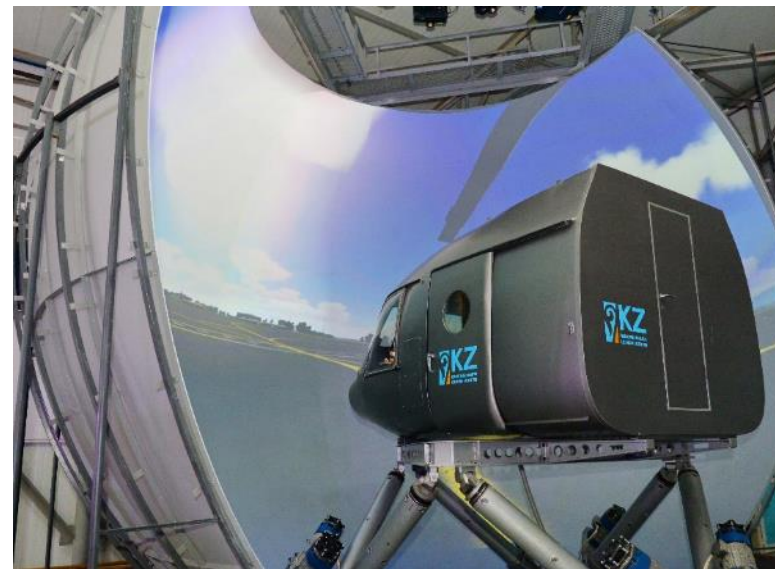
Динамический тренажер экипажа вертолета Ми-17
